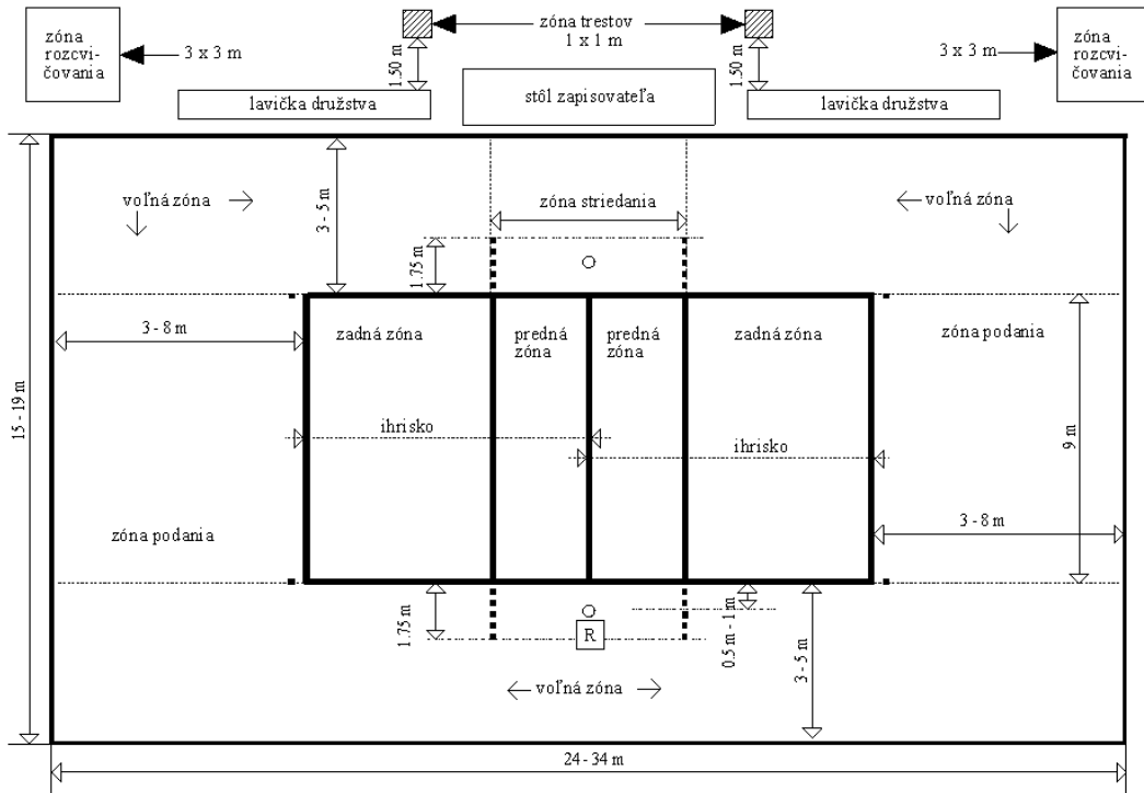
Obr. 1. Hracia plocha (pravidlo 1, 1.4.2)
